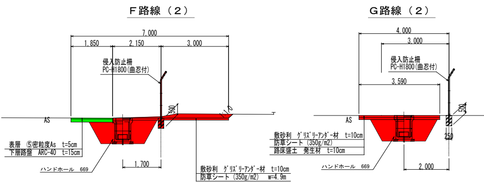
【標準横断図F・G】
