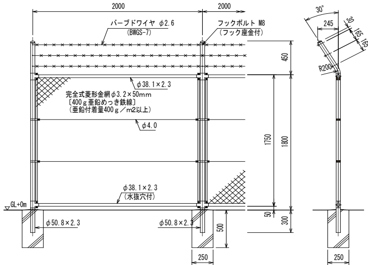
【標準横断図F・G】
